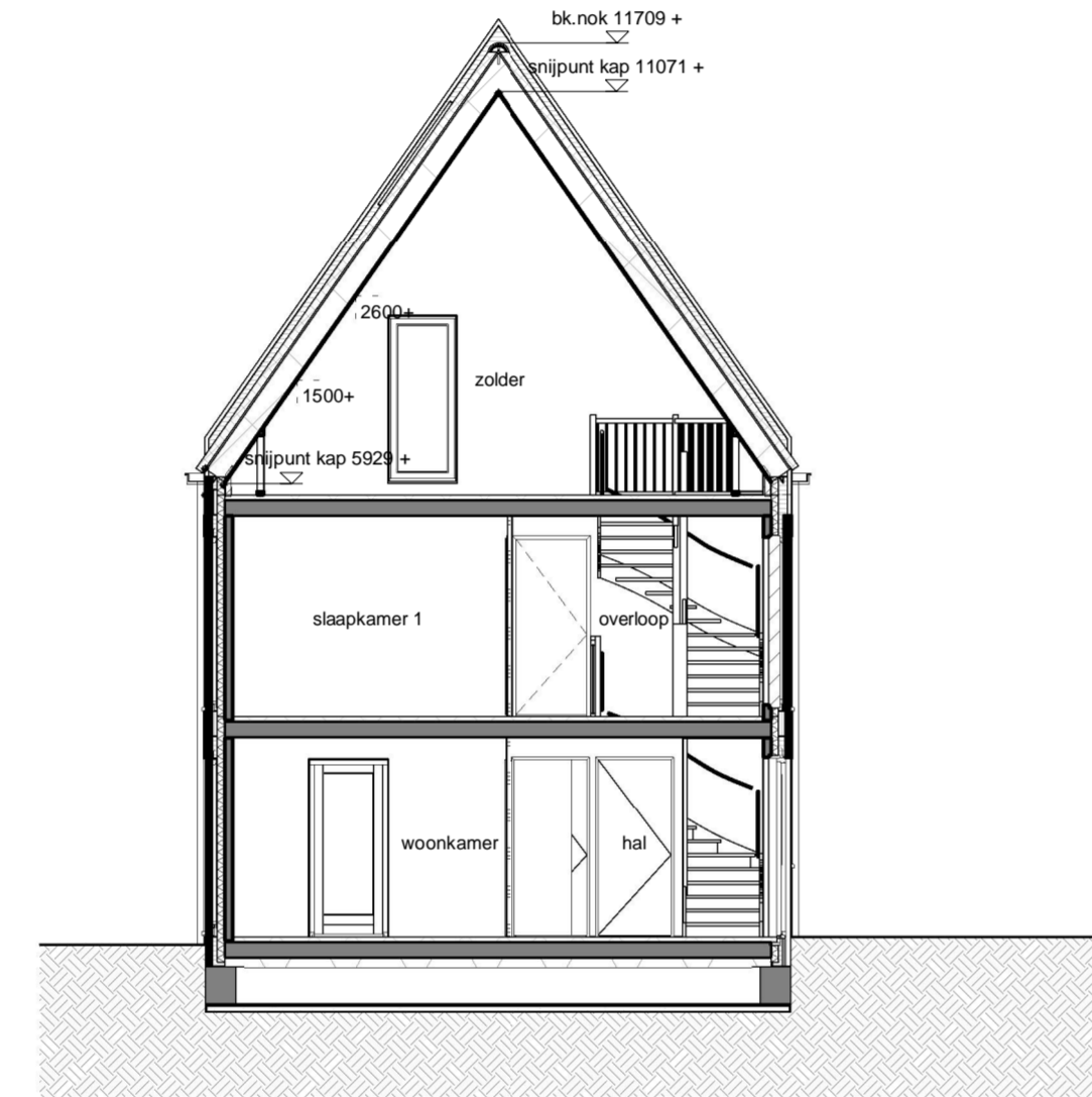
Dwarsdoorsnede
