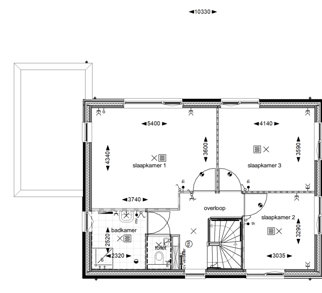
Eerste verdieping
