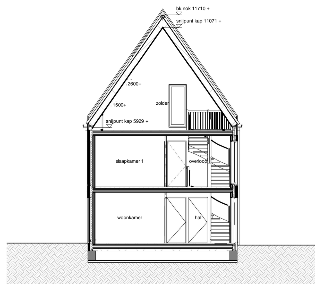
Dwarsdoorsnede
