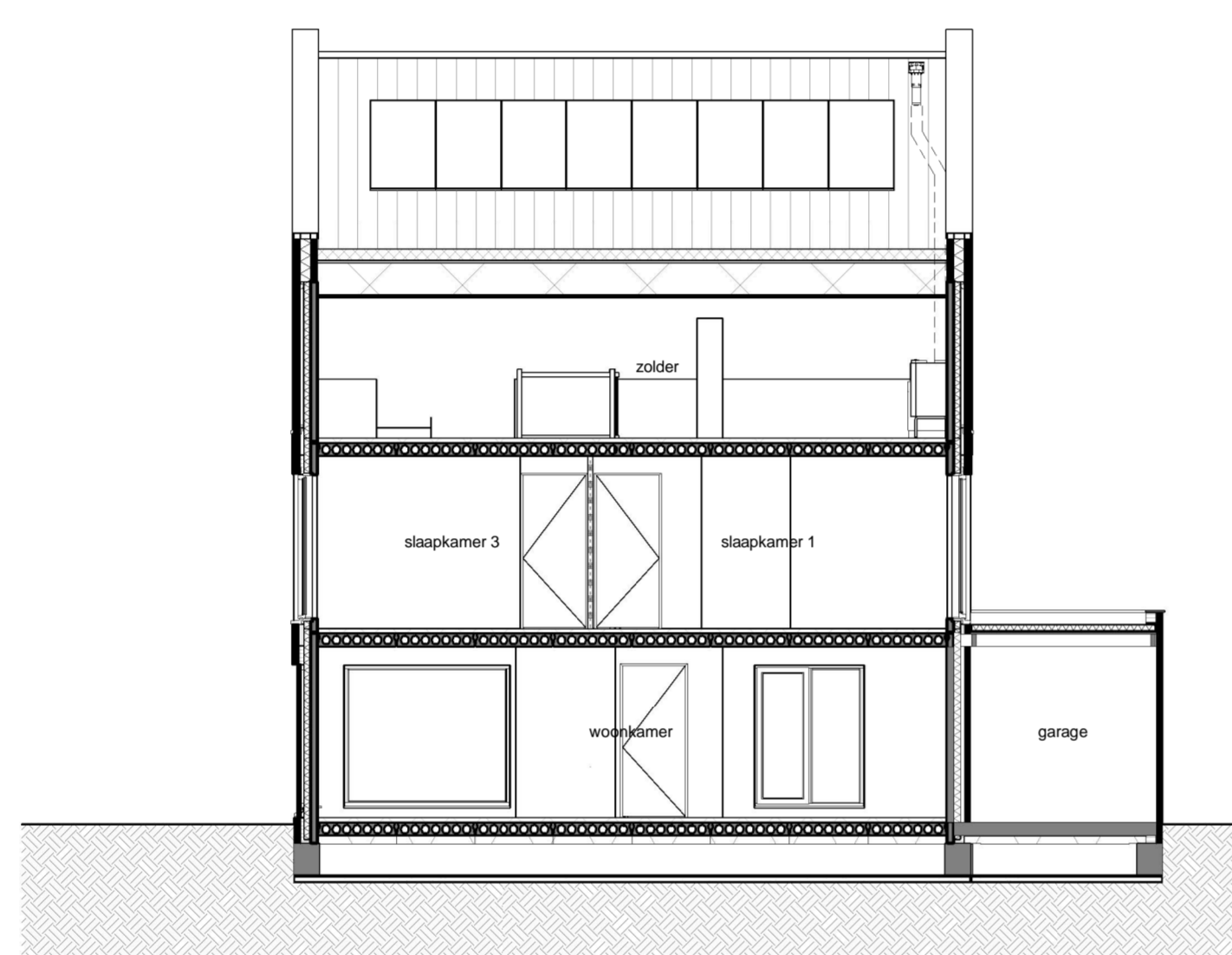
Langsdoorsnede
